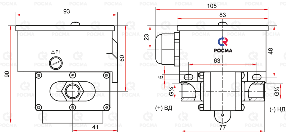
РДД-2Р с внутренней резьбой G \frac{1}{4}
