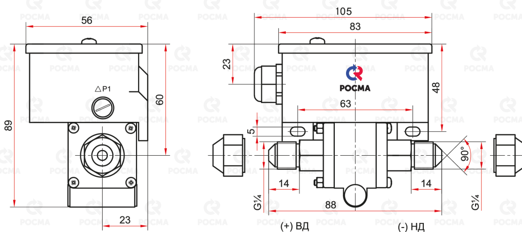
РДД-2Р с наружной резьбой с накидной гайкой G \frac{1}{4}
